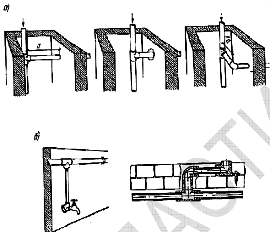
Рис.26. Прокладка пластмассовых труб:
