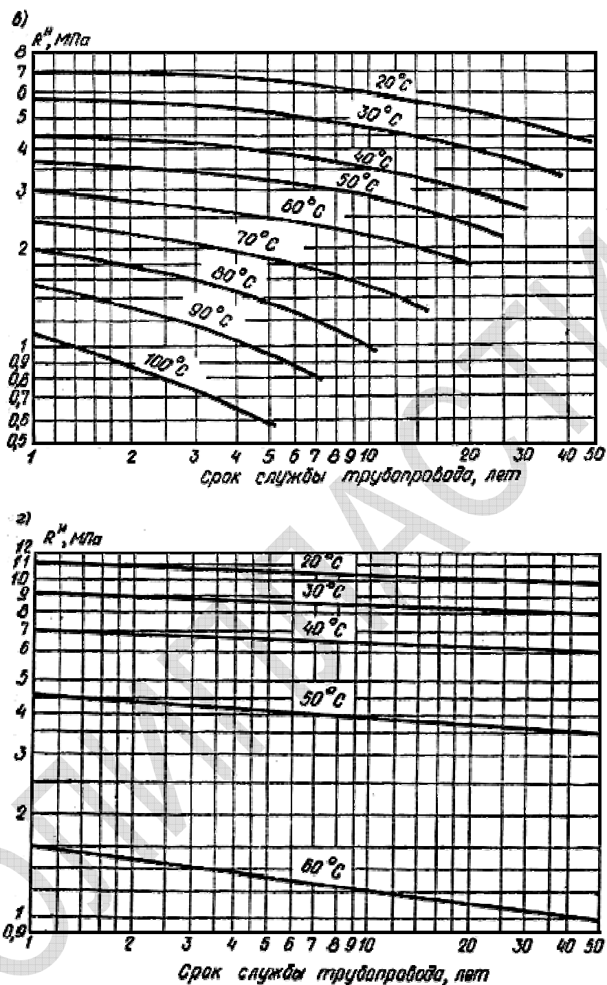
Рис.1. Зависимость нормативного длительного сопротивления разрушению R_H материала труб от температуры и срока службы трубопровода для труб:
