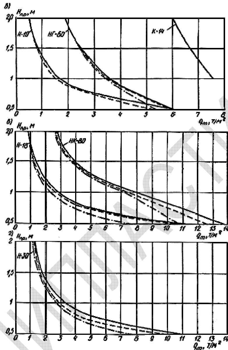
Рис.41. Зависимость нормативного давления от транспорта q_{тр}^к , от глубины заложения трубопровода H_{пр} при диаметре труб 110 мм (сплошные линии), при диаметре труб 50 мм (пунктирные линии) и при диаметре труб 1200 мм (штрихпунктирные линии):
