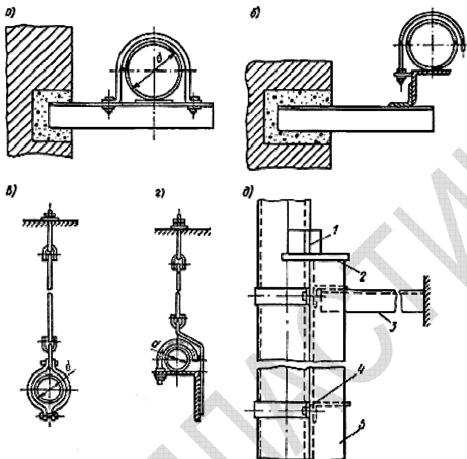
Рис.39. Опоры и подвески по ОСТ 36-17-77:
