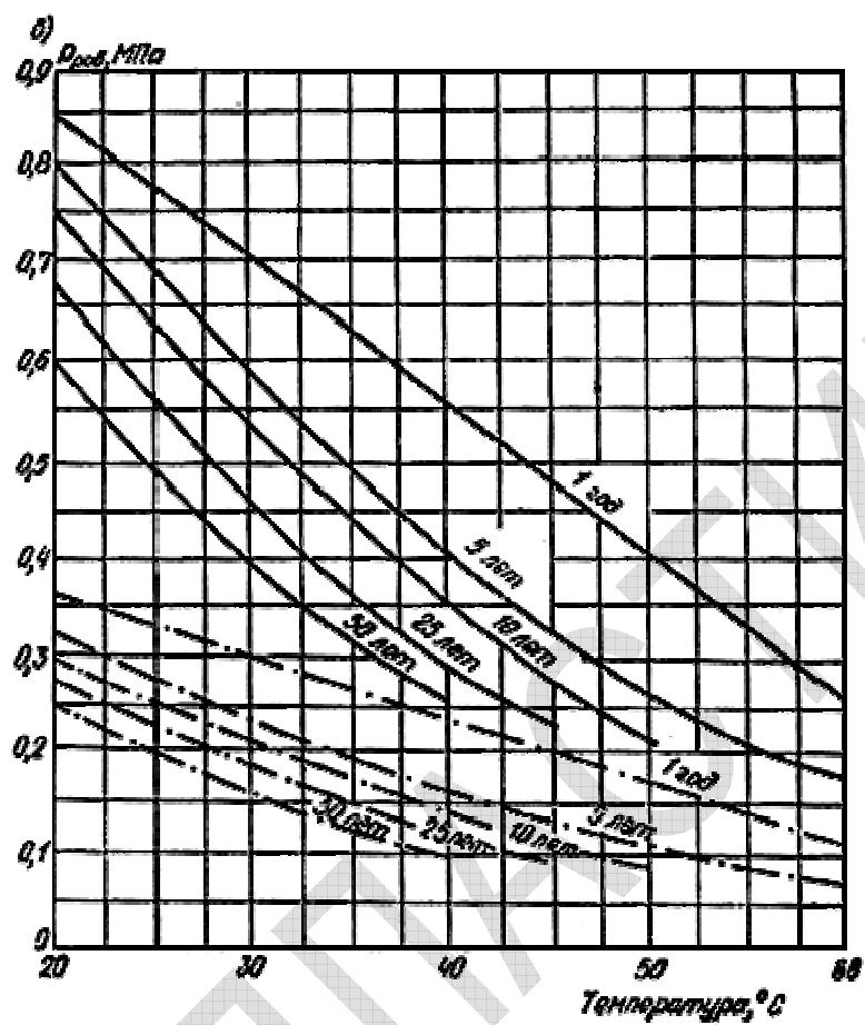
Рис.2. Зависимость рабочего давления P_{раб} от температуры и срока службы трубопровода для труб из ПНД:
