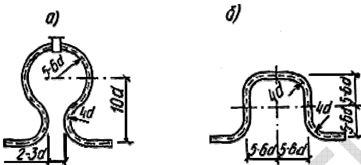
Рис.28. Компенсаторы для трубопроводов из ПВХ:
