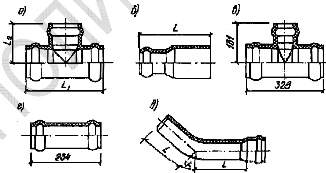
Рис.16. Соединительные детали из ПВХ для раструбных труб:
