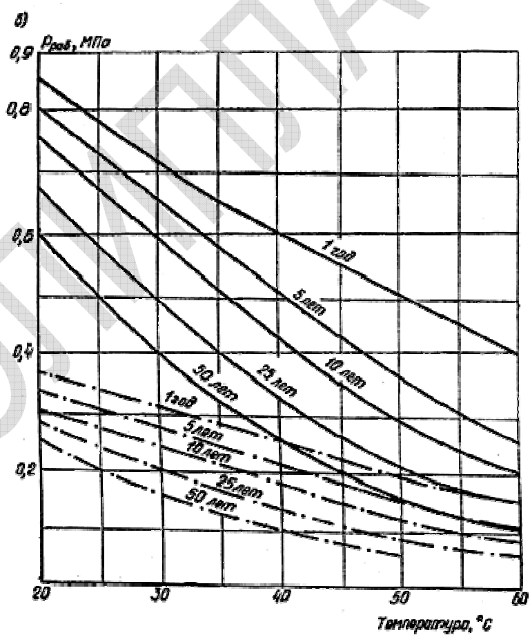
Рис.3. Зависимость рабочего давления P_{\text{раб}} от температуры и срока службы трубопровода для труб из ПВД:
