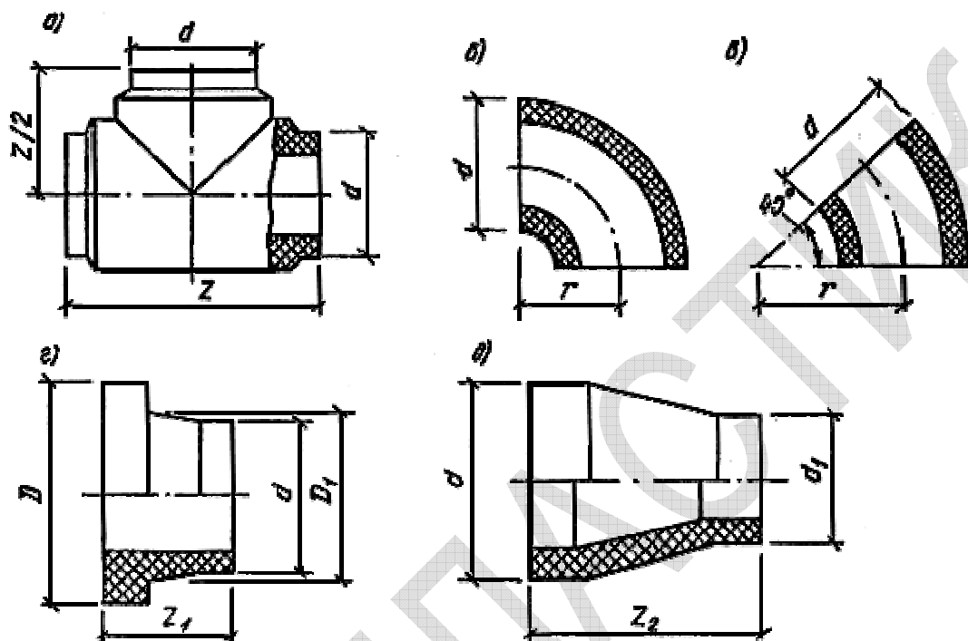
Рис.11. Соединительные детали из ПНД, изготавливаемые методами литья под давлением, прессованием и намоткой:
