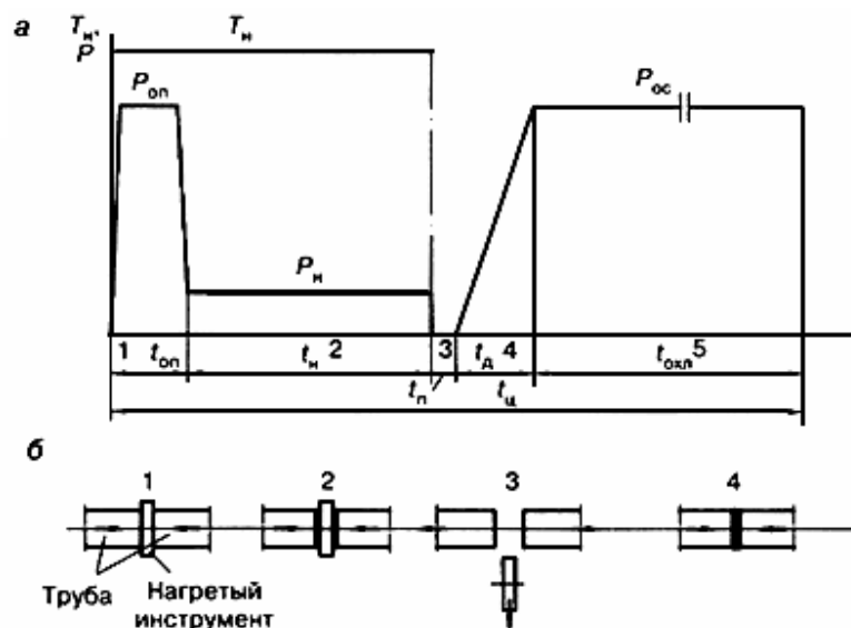
а - диаграмма изменения во времени t давления на торцах P и температуры нагретого инструмента T_H ; б - последовательность протекания процесса сварки;
