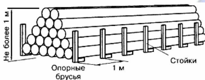
Рисунок 9 - Хранение отдельных труб в штабеле
