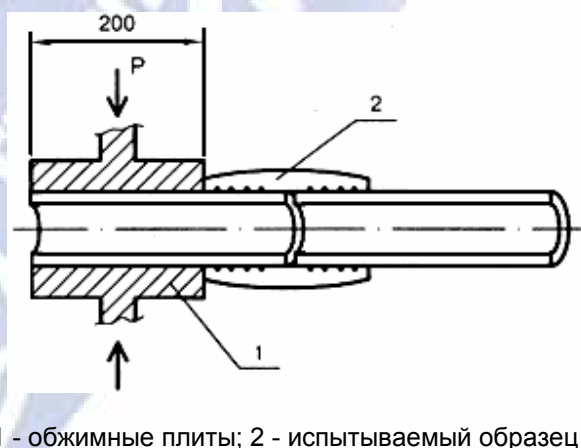
Рисунок Т.2 - Схема испытания образцов-сегментов на сплющивание
