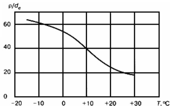
Рисунок 18 - Зависимость отношения радиуса упругого изгиба газопроводов \rho к наружному диаметру трубы d_g от температуры окружающего воздуха T при монтаже и укладке газопроводов
